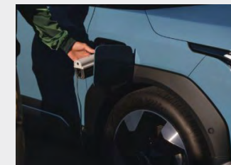
Connettore V2L esterno
